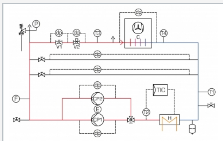
Esquema del proceso: dp presión diferencial, F caudal, T temperatura, E potencia eléctrica, TIC regulación de temperatura, C convector, H dispositivo de calefacción, CP bomba de circulación, V1 válvula de equilibrado, V2 válvula de termostato
