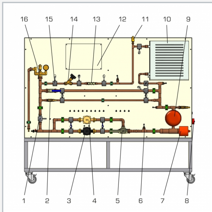
1 sensor de caudal, 2 válvula, 3 bomba convencional, 4 bomba regulada por presión diferencial, 5 llave esférica de tres vías, 6 sensor de temperatura, 7 dispositivo de calefacción regulable, 8 paro de emergencia, 9 vaso de expansión, 10 convector, 11 ventilador, 12 esquema de proceso, 13 válvula de termostato, 14 válvula de equilibrado, 15 punto de medición de presión diferencial, 16 grupo de seguridad de la
